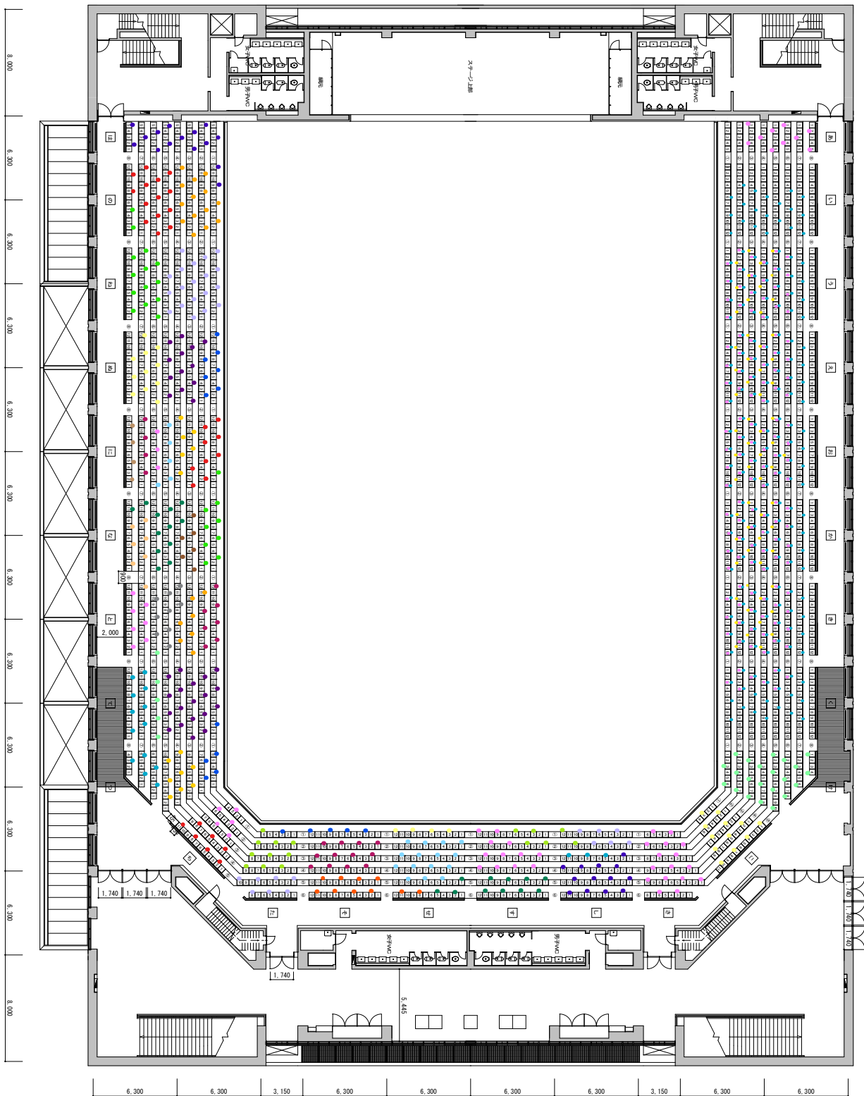
高松市総合体育館 第1競技場2階平面図 S=1/200
