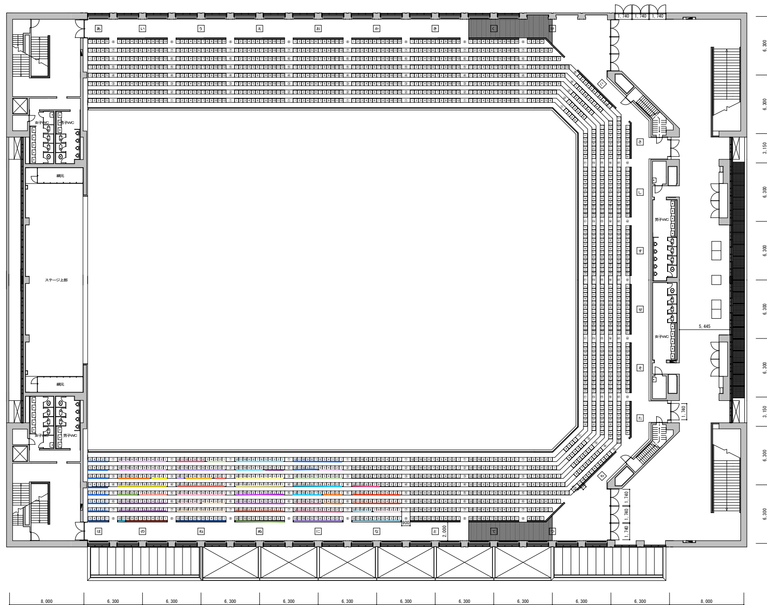
高松市総合体育館 第1競技場2階平面図 S=1/200
